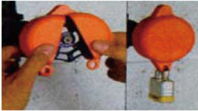
㉠ 커버용 잠금장치
